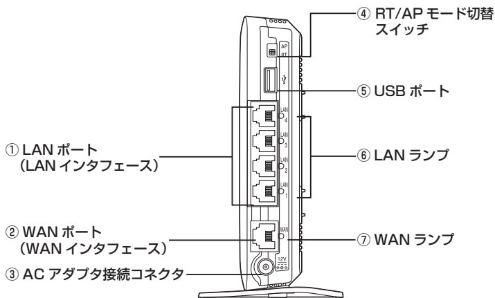
〈背面〉
